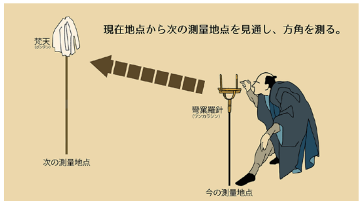
▲彎窠羅鍼（わんからしん）を使った測量風景（模式図）
