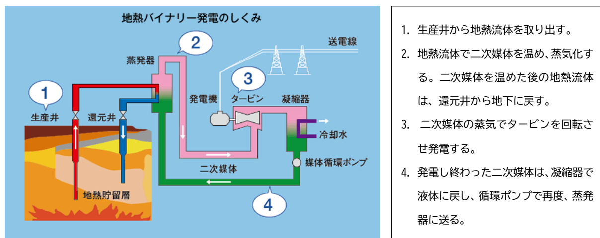
図 6-7 地熱バイナリー発電の仕組み 出典: 日本地熱協会「地熱発電のしくみ」
