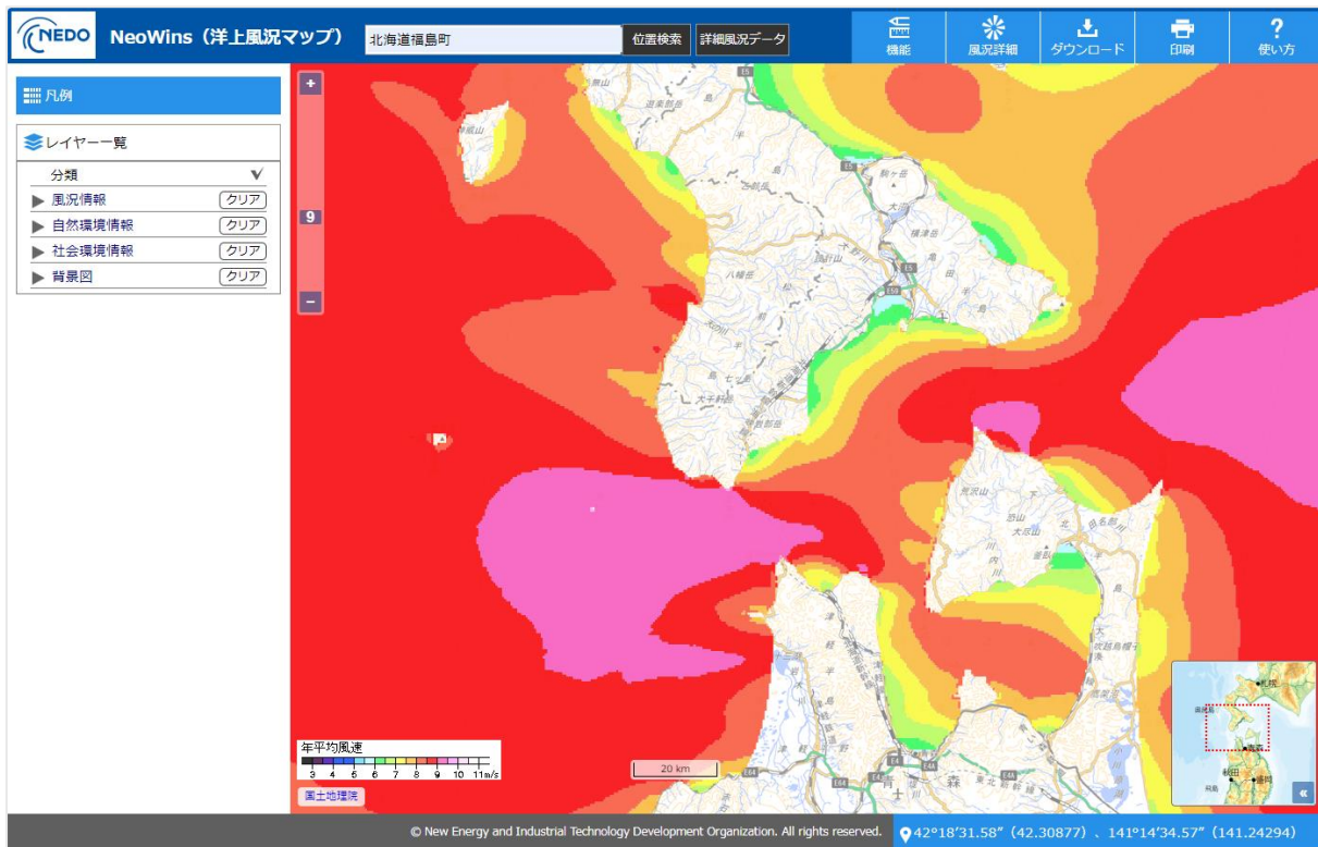
図 2-10 福島町および周辺地域の年平均洋上風速 出典:NEDO「NeoWins(洋上風況マップ)」
