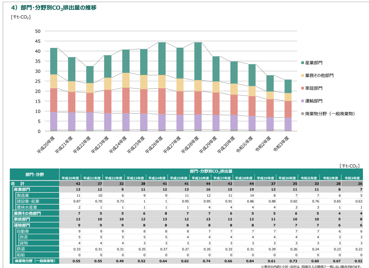
図 4-1 福島町の「自治体排出量カルテ」(令和 6 年 3 月)における部門・分野別 CO 2 排出量の推移
