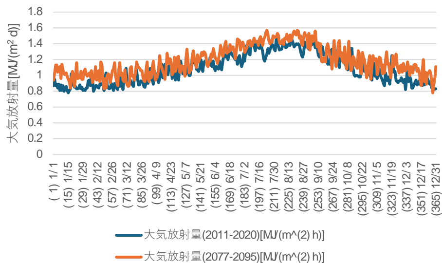
図 9-7 現在の標準気象データと 2080 年代標準気象データの大气放射量の比較
