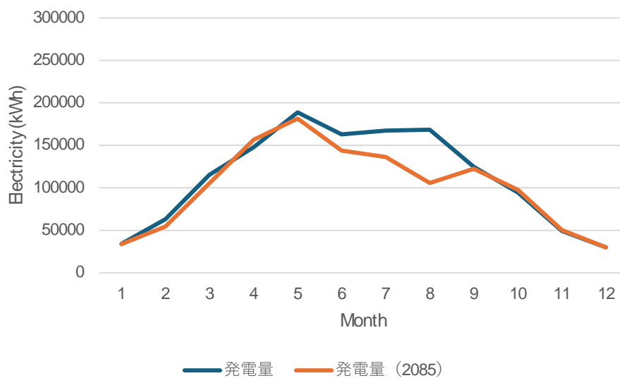
図 9-10 水平設置の場合の発電量
