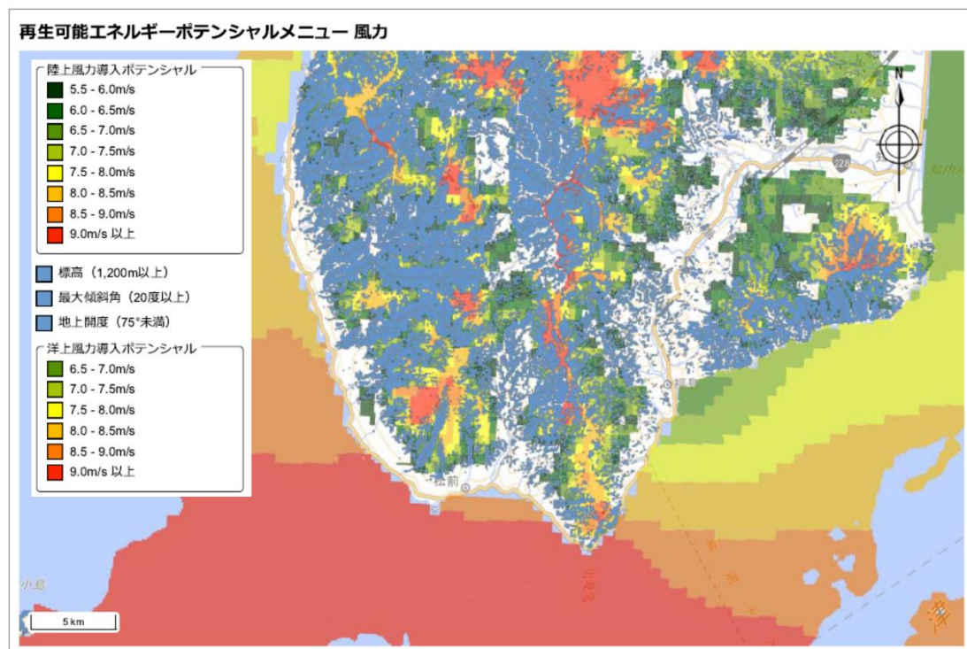
図 7-8 風力発電の導入ポテンシャル(福島町)
