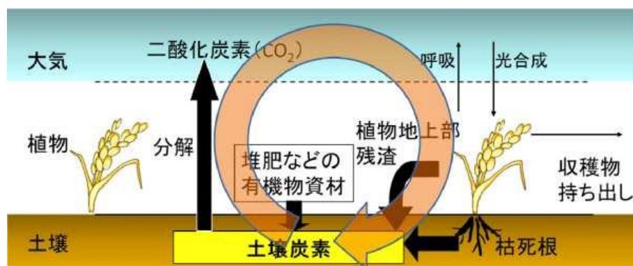
図 6-22 土壌の炭素循環
