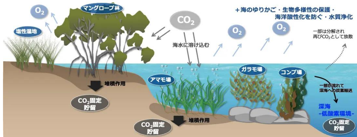
図 6-23 ブルーカーボンのメカニズム
