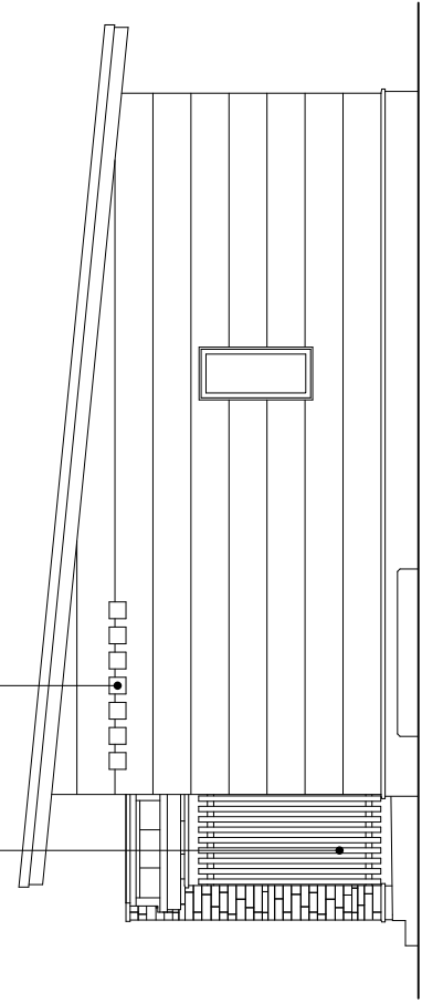
西立面図
