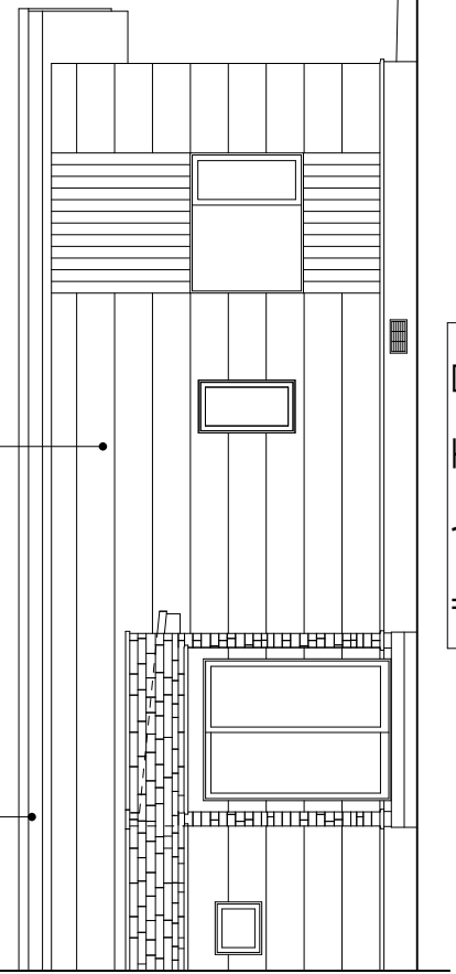
北立面図
